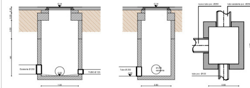
PARTICOLARE POZZETTO 80x100 (N. 3) - scala 1:20
