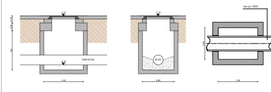
PARTICOLARE POZZETTO 80x100 (N. 4) - scala 1:20
