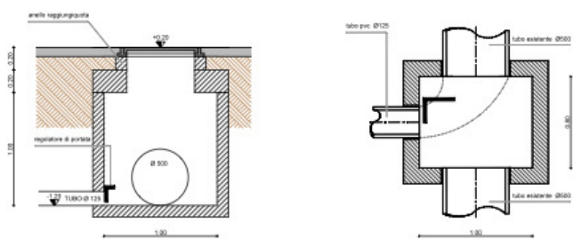
PARTICOLARE POZZETTO 80x100 (N. 4) - scala 1:20
